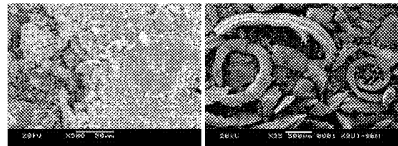
(c) Fe/Sn film/Fe (d) Fe/Sn-Al 2 O 3 film/Fe
