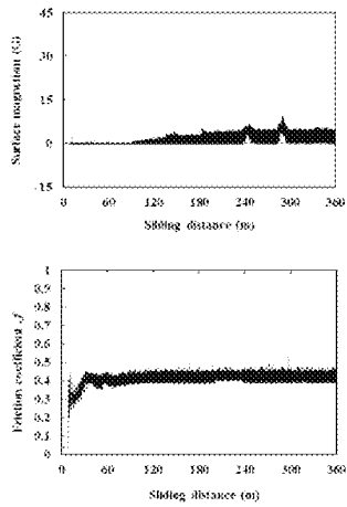
圖 7 CrO 2 在 80N 及 200mm/s 條件下之動態摩擦係數與表面磁場的響應
