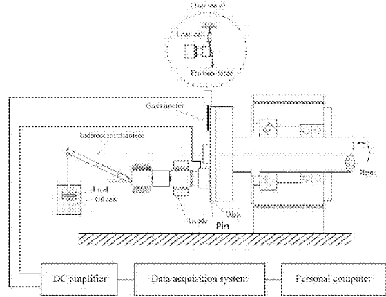
圖 1 旋轉式摩擦磁化試驗機暨量測系統
