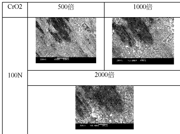
圖 10 CrO 2 在 100N 及 200mm/s 條件下之 SEM 圖
