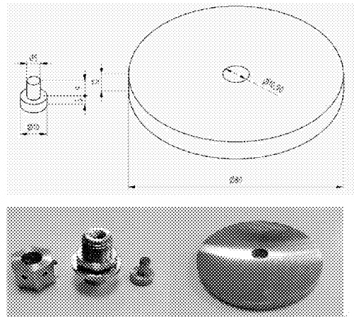
圖 3 實驗試片及尺寸
